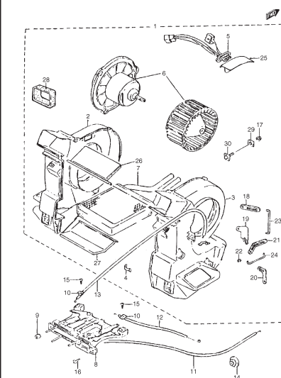
FIG. 78 HEATER
