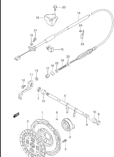
FIG. 23 CLUTCH
