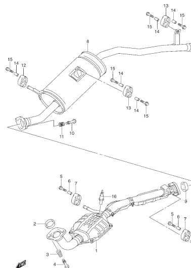
FIG. 16 MUFFLER
