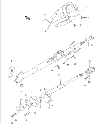
FIG. 54 STEERING SHAFT
