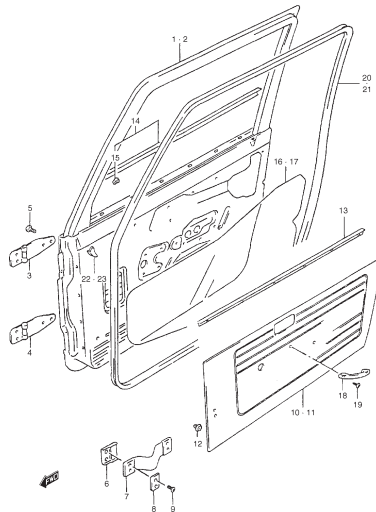
FIG. 86 FRONT DOOR PANEL
