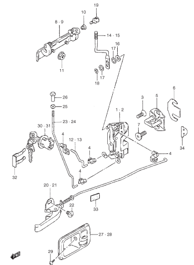
FIG. 88 FRONT DOOR LOCK
