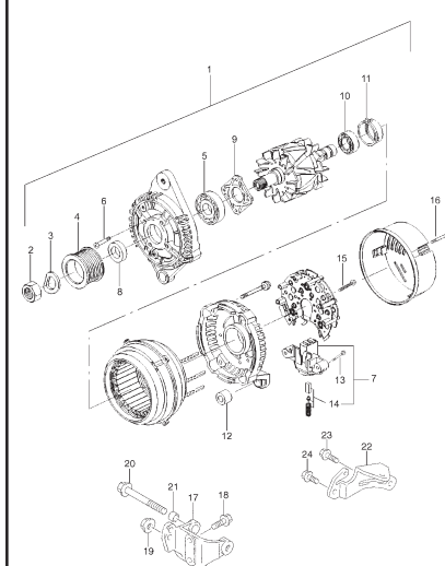
FIG. 36 GENERATOR
