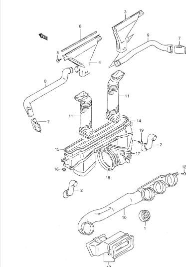
FIG. 77 VENTILATOR
